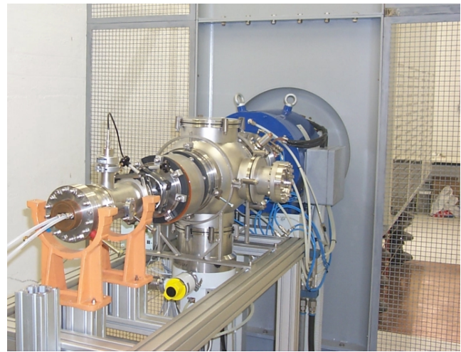
Figure 8: The LEBT line.
