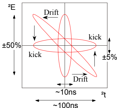
Fig. 1 Phase rotation technique.
