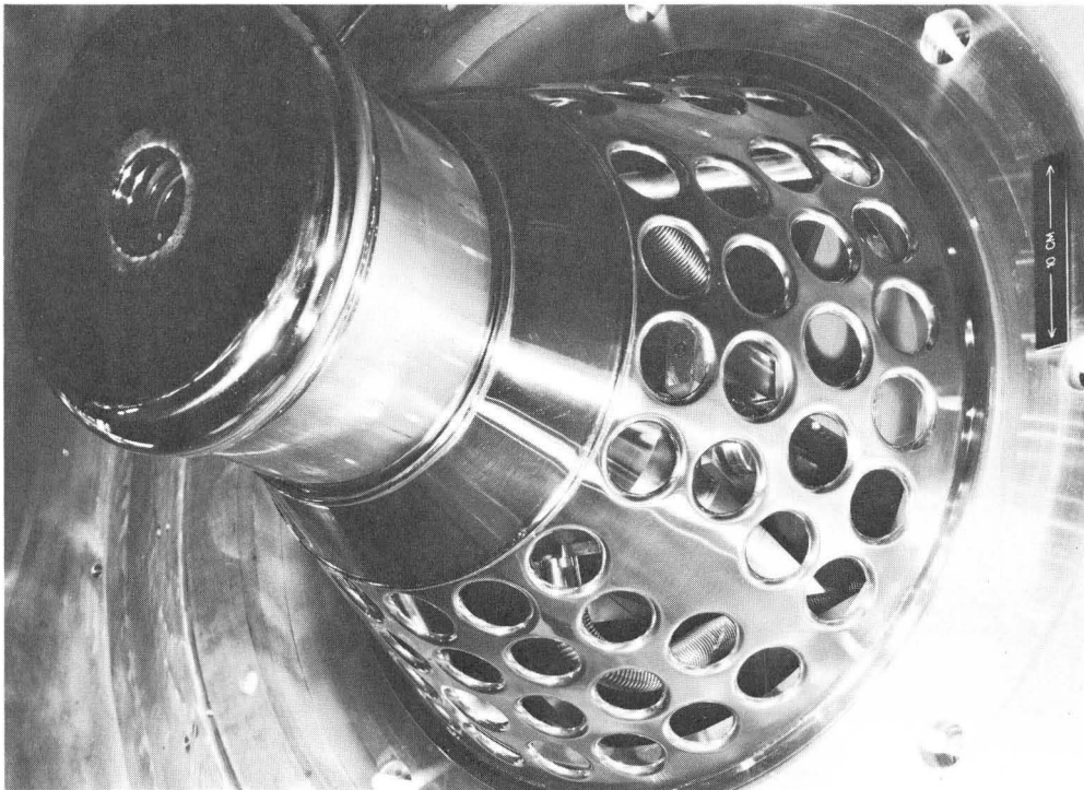
Fig. 5 Titanium alloy cathode.
