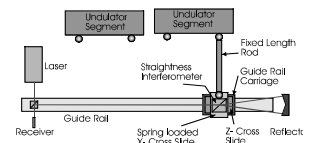
Fig. 4 Interferometer
