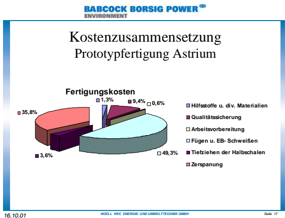
Fig. 1: Relative costs of the cavity prototype production at Astrium. (Hilfsstoffe u. div. Material: auxiliary material; Qualitäts-sicherung: quality assurance; Arbeitsvorbereitung: preparation of working steps; Fügen u. EB Schweißen: assembly of parts and EB welding; Tiefziehen der Halbschalen: deep drawing of cups; Zerspanung: cutting and milling)
